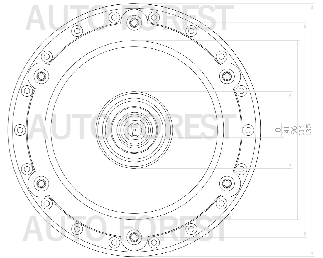
Right view Scale: 1:1
